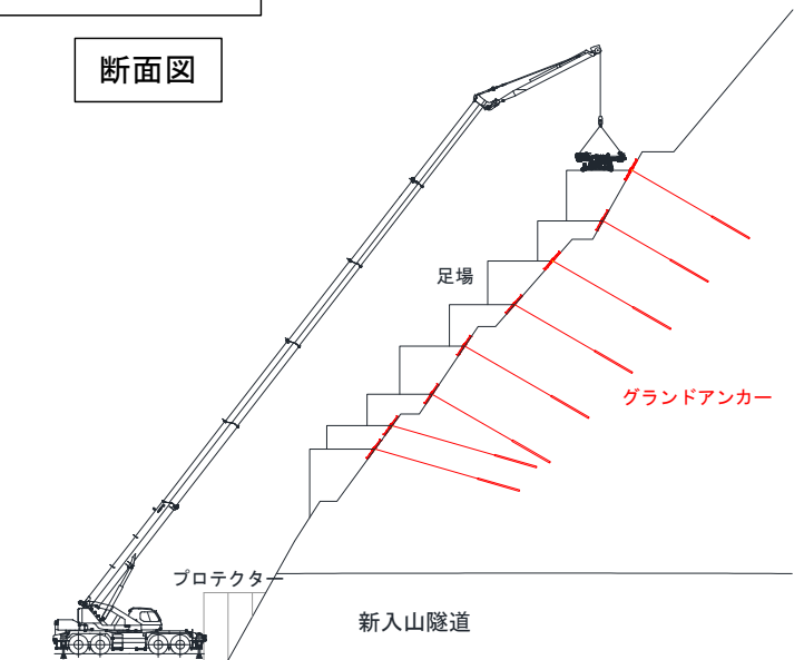
グラウンドアンカー設置状況
